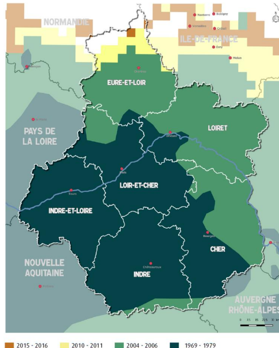
Evolution temporelle du front de colonisation de la chenille processionnaire du pin, Centre-Val de Loire
