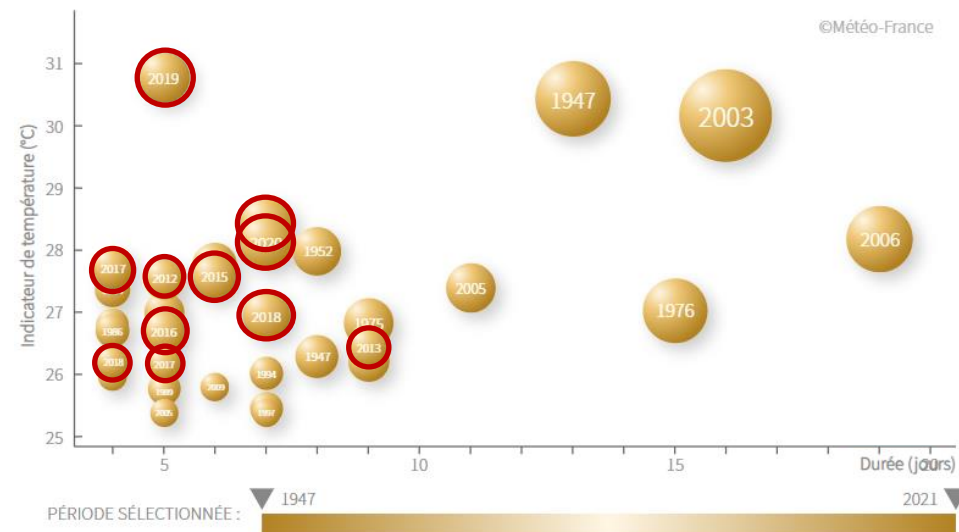
Evolution des vagues de chaleur, période 1947-2021, région Centre-Val de Loire
