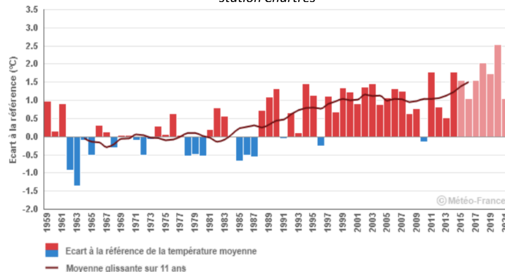
Températures moyennes annuelles : écart à la référence 1961-1990, station Chartres
